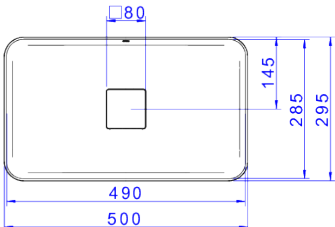
Desenho Técnico
